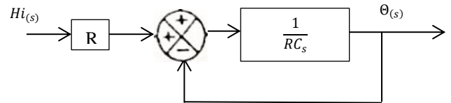
Gambar 4. Diagram kotak sistem pemanas inkubator
