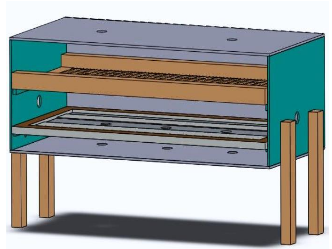
Gambar 3. Desain Mesin Tetes Telur
