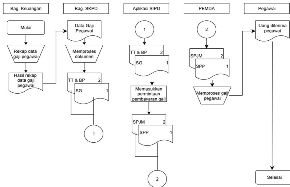
Gambar 2. Flowchart Sistem Informasi Pemerintahan Daerah (SIPD)
